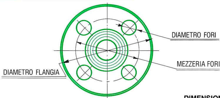
DIMENSIONI DELLE FLANGE UNI
